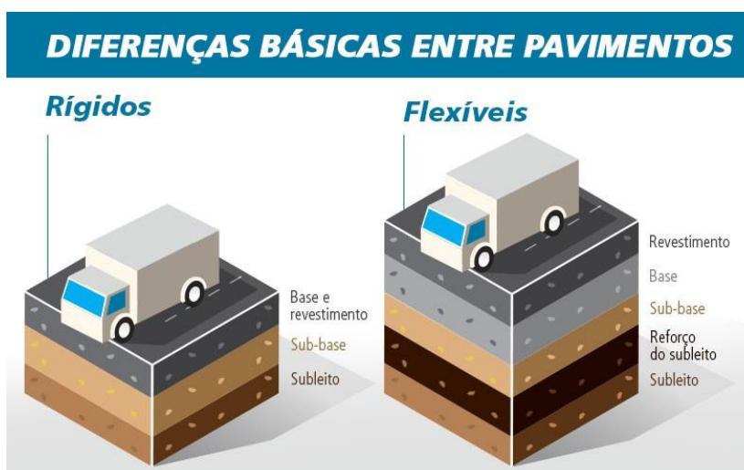
Figura 1 – Camadas Pavimentação Rígida - Fonte: Votorantim Cimentos – Mapa da obra
