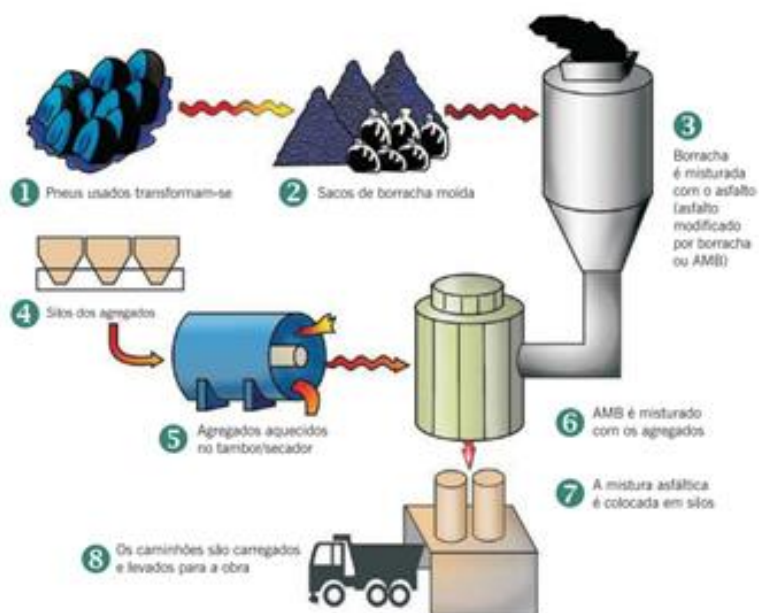
Figura 3 Esquema de fabricação do asfalto-borracha via úmida pelo processo de mistura – Fonte: Bernucci (2008)
